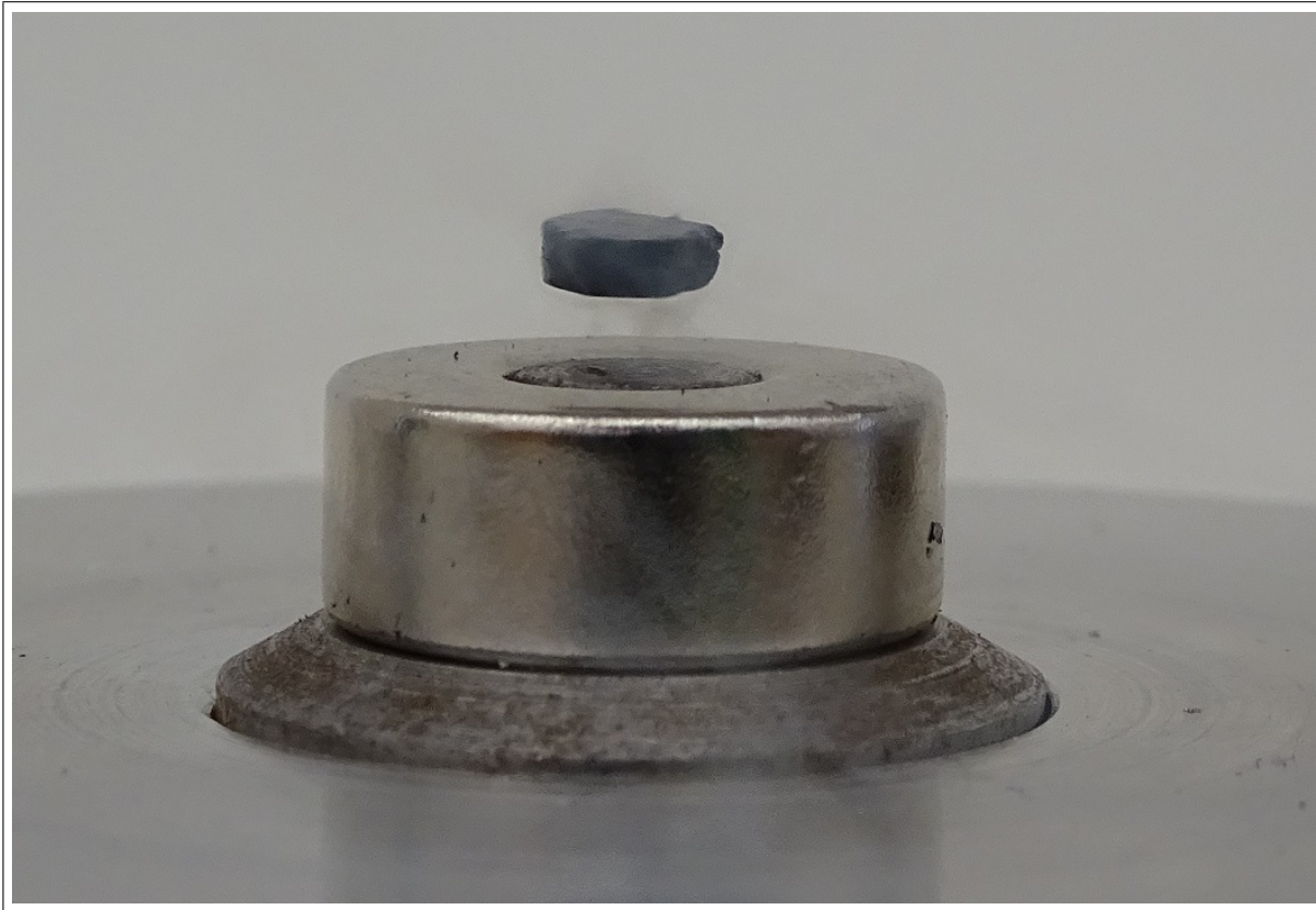
Abbildung 2: Schwebender Supraleiter
