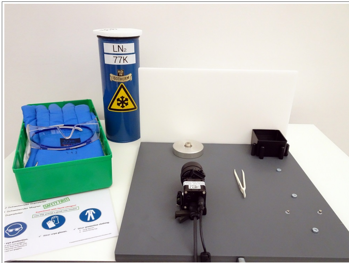
Abbildung 1: Versuchsaufbau „Schwebender Supraleiter – Meissner-Effekt“
